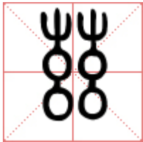
兹字的篆书
