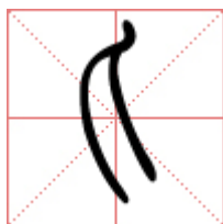
匕字的篆书
