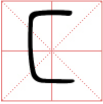
匚字的篆书
