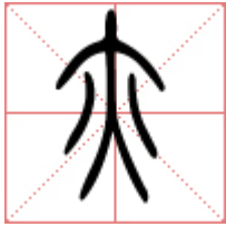
腋字的篆书
