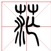
茫字的篆书
